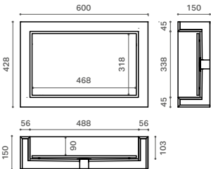
60×42,8 cm scarico nascosto/concealed drainage
